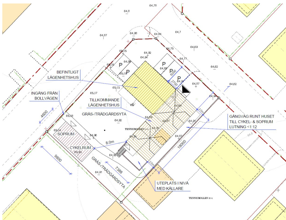
Figur 4 Situationsplan utvecklingsförslag.
