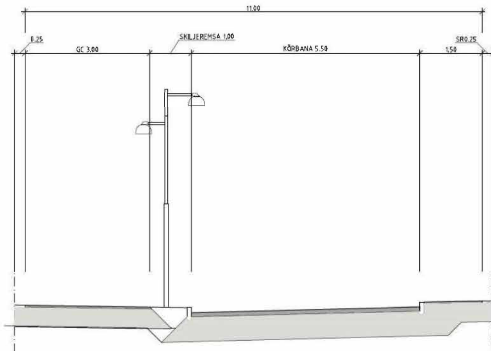
Typsektion för Trollskogsgatans förlängning
