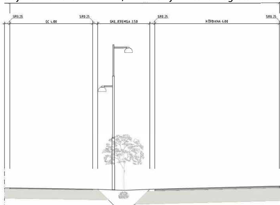
Typsektion för den öst-västliga gatusträckan, benämnd som genomfartsgataovan
