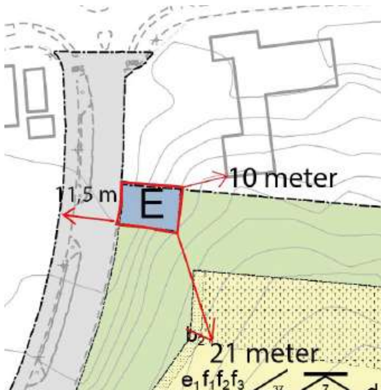
Illustration med avstånd norra E-området invid Trollskogsgatan
