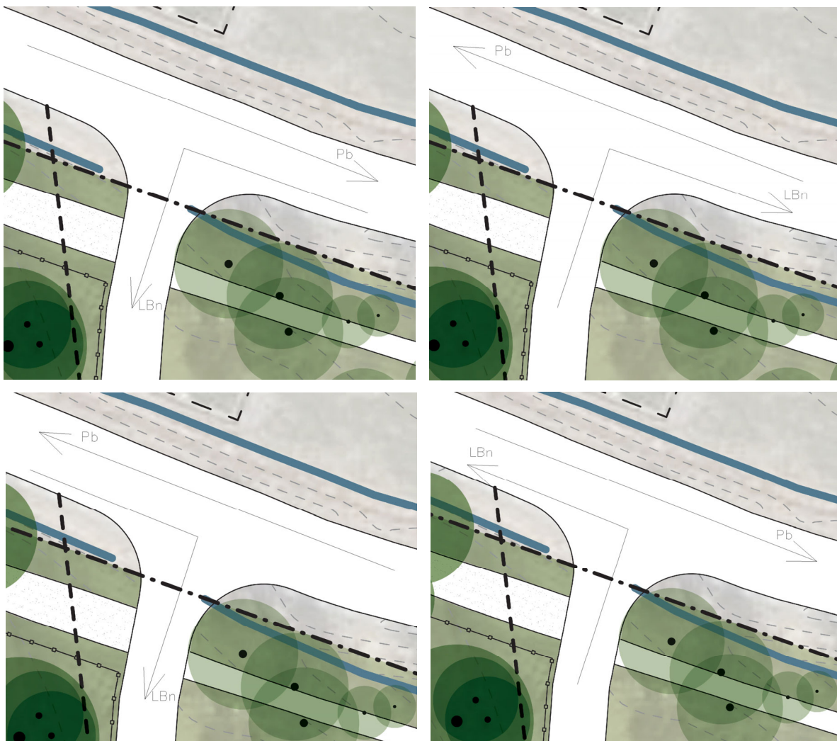
Figur 11 Infartsvägens dimensionering med personbilarnas möte med lastbil (12 meter) på Kärrbogärdevägen.
