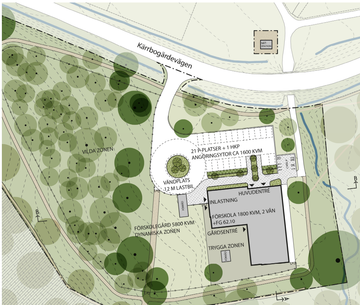
Figur 10 Situationsplan för förskolan. Underlag framtaget av Krook & Tjäder.
