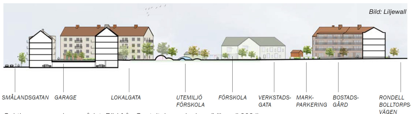
Sektion genom planområdet. Bild från Gestaltungsprinciper (Liljewall 2024).
