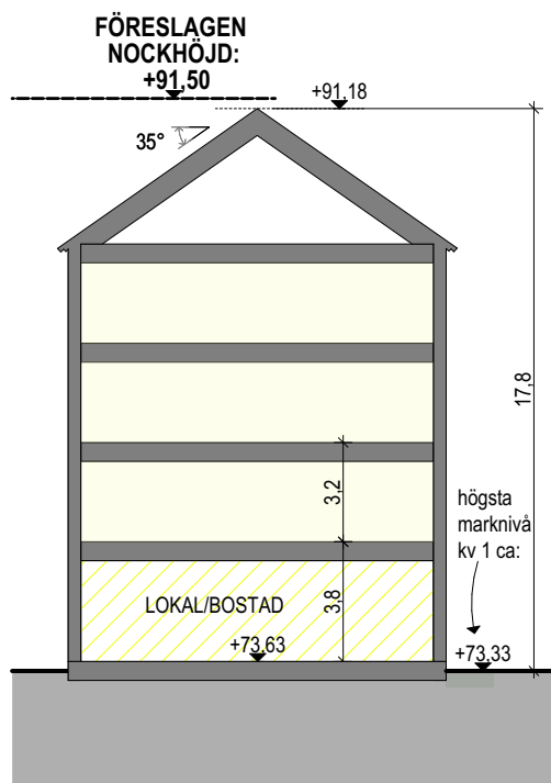
Underlag till nockhöjder, sektion över kvarter 1, till vänster, respektive kvarter 4 till höger (Liljewall 2023).
