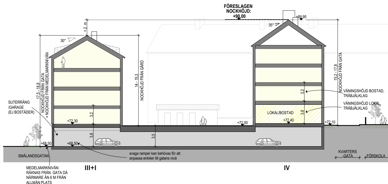
Underlag till nockhöjder, sektion över kvarter 2 och 3, längs med Smålandsgatan (Liljewall 2023).
