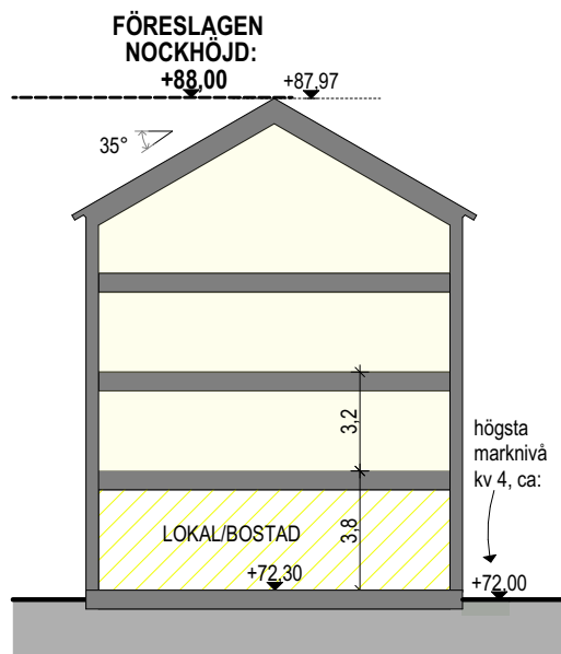
Underlag till nockhöjder, sektion över kvarter 1, till vänster, respektive kvarter 4 till höger (Liljewall 2023).
