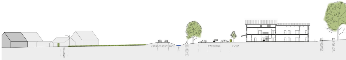
Figur 8. Marksektion A-A – nord-sydlig riktning.
