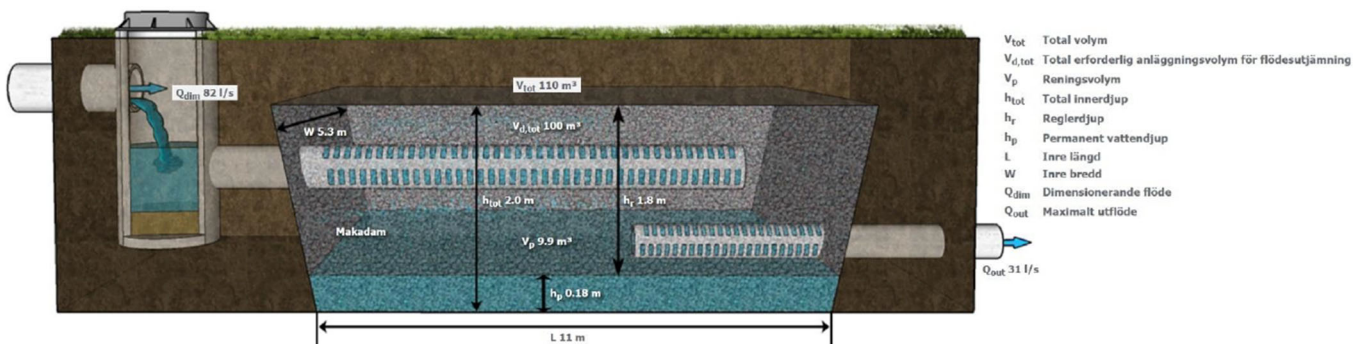
Figur 16. Makadammagasinet's fördröjningsvolymers, ytanspråk och utformning (Rejlers 2024).
