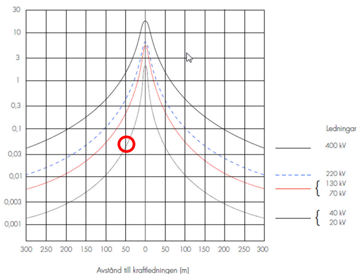
Figur 32. Diagrammet visar magnetfältets styrka på olika avstånd från luftledningar med olika spänningsnivåer. Röd markering redogör för magnetfältets styrka på ett avstånd om 50 meter. Illustration: Strålsäkerhetsmyndigheten.
