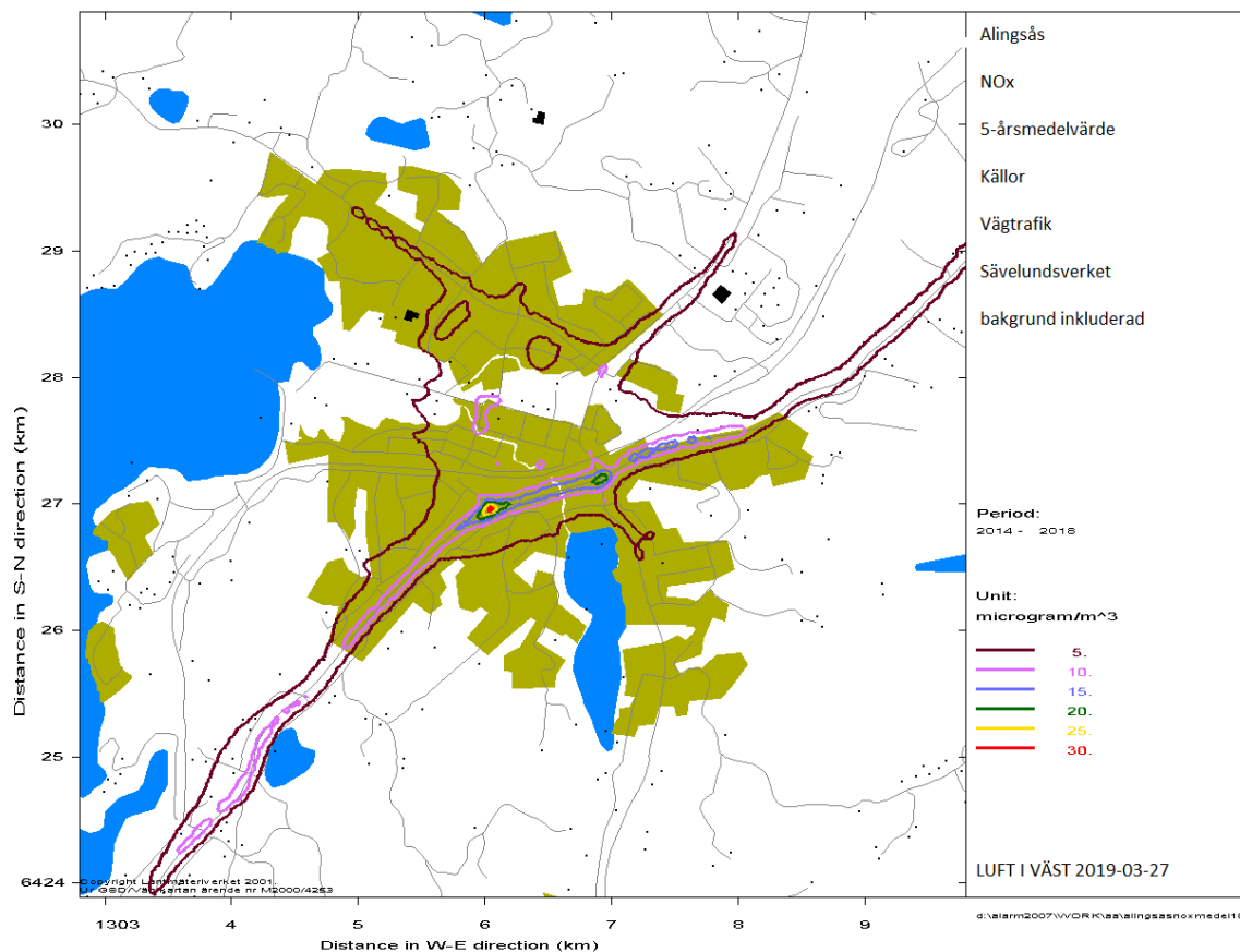
Figur 1 Resultat av en spridningsberäkning av årsmedelvärden kväveoxider (kväveoxid + kvävedioxid) i Alingsås tätort baserat på data från perioden 2014–2018. Modellsystem: ALARM.
