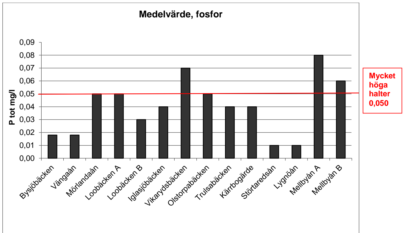
Diagram 3. Medelvärdesberäkningar av fosforkoncentrationen, höga halter för P_{tot} > 0,025 mg/l och mycket höga halter > 0,05 mg/l (Naturvårdsverkets bedömningsgrunder, 1999).
